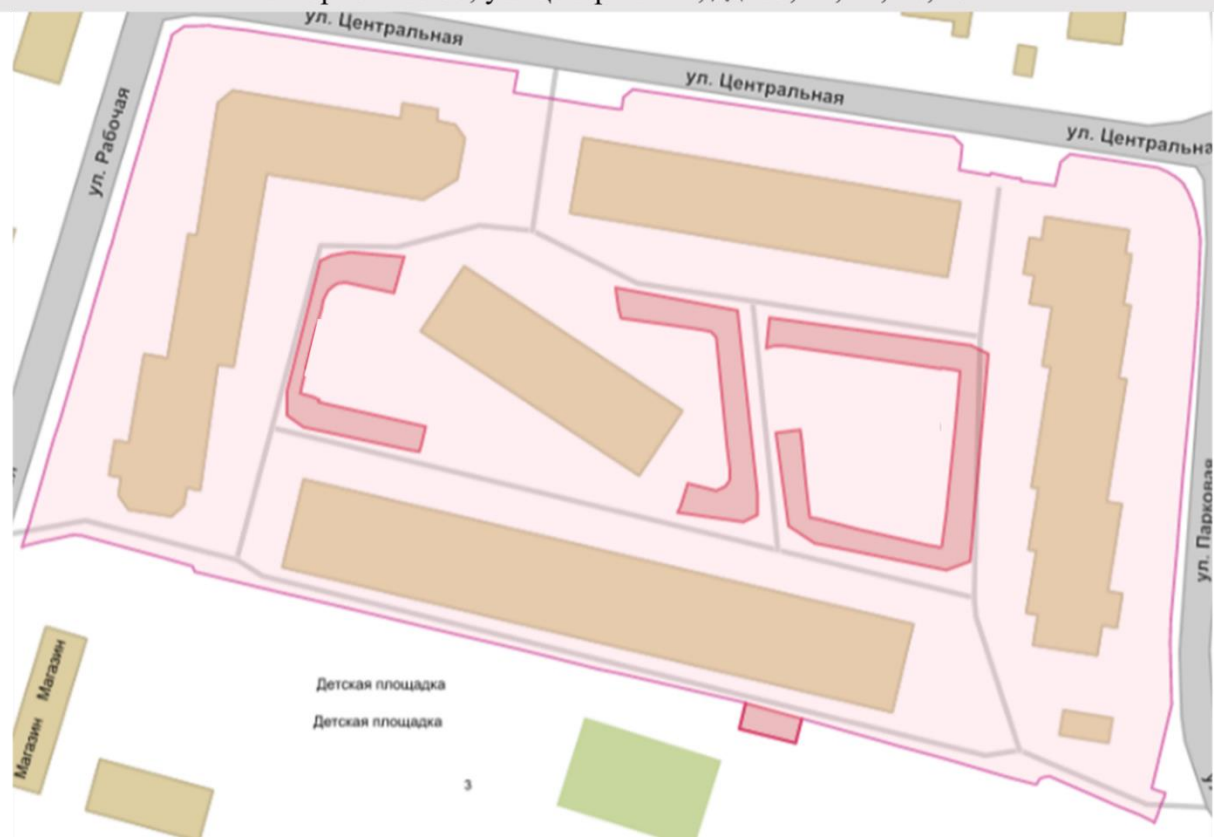
Схема расположения плоскостных сооружений дворовой территории п. Первомайское, ул. Центральная, дд. 18, 22, 24, 26, 27
